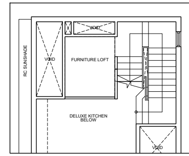
LOFT - PLAN
