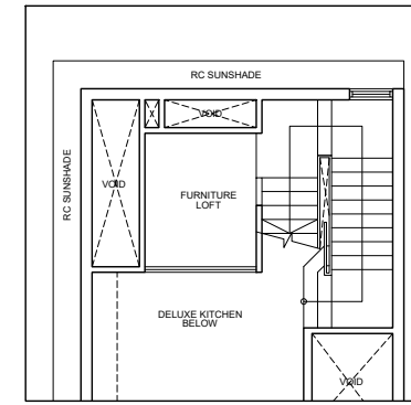
LOFT - PLAN
